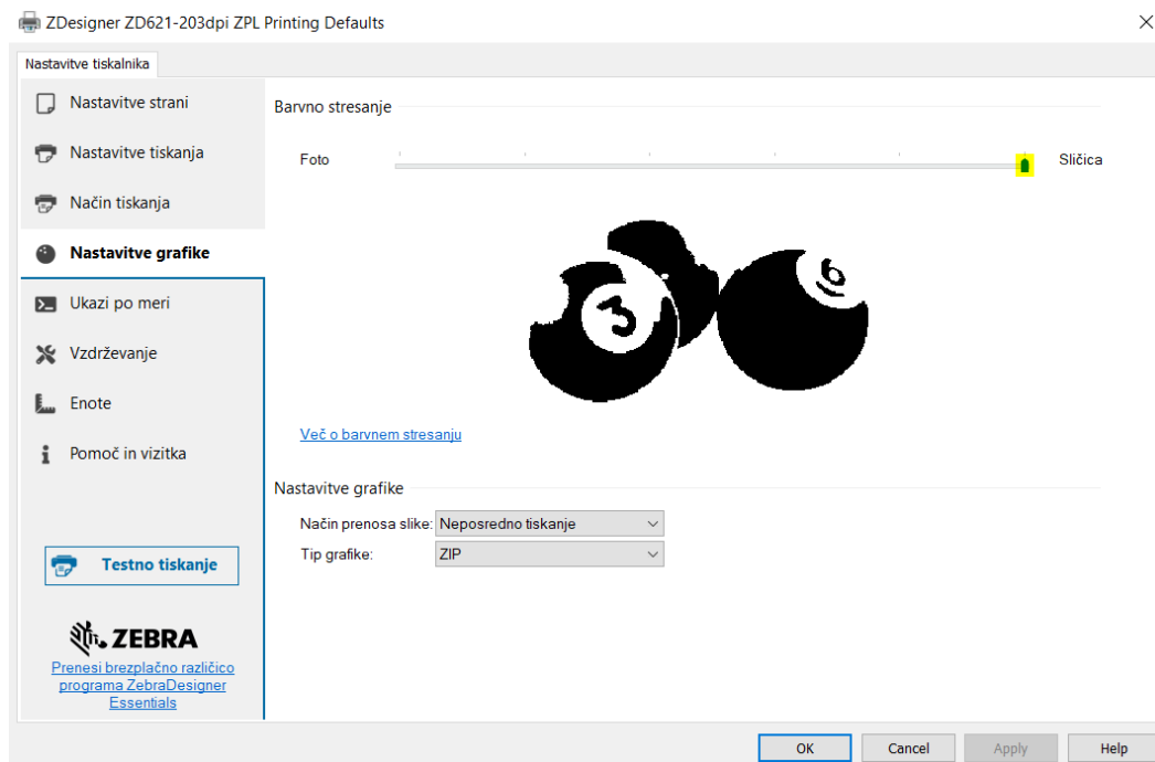
Slika 7: Nastavitve grafike
